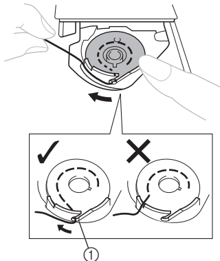
① 장력 조절 스프링
